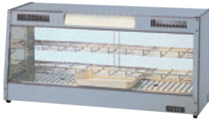
⑤ ホットショーケース NH-403 H-10 直 / 元払・1台 寸法:900×300×415 / 100V・740W 1台 ¥169,000 611-3402 棚板2段可変 ケース内は50~80℃まで温度調節自由自在 耐久性に優れたステンレス製
