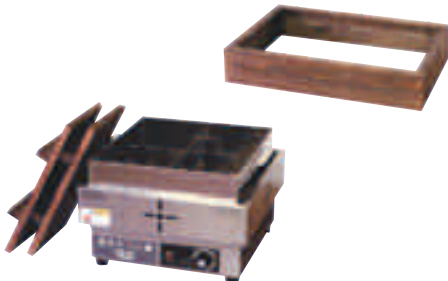
⑦ 電気おでん鍋 H-10 直 / 元払・1台 規格 寸法 内容積 1台 NHO-4SY 340×335×277 11.1ℓ ¥106,000 612-6004 4SY用木枠 373×368×105 ¥ 13,100 612-6005 100V・670W / 可変式サーモスタット 使用温度範囲:70℃~100℃ ステンレス製 / 鍋と仕切り枠は取り外し可
