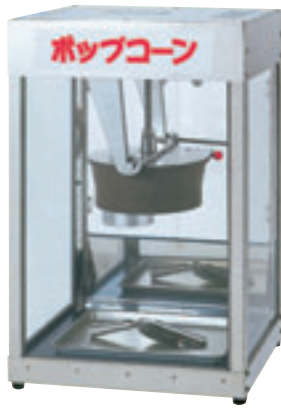
①ポップコーン機 POP-8F N-6 直 /元払・1台 寸法・470×400×715 / 100V・1210W 1台 ¥280,000 611-6608 能力・3分毎に280g(六角カップ8杯、三角カップ11杯)
