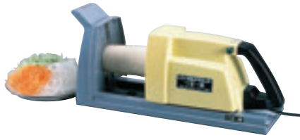
② 電動ツマカッター HS-010 N-6 在 寸法・470×160×220/100V・80W 1台 ¥108,000 611-0010 標準セットクシ刃 1.2mm 処理能力・大根50~100本/時 HS-112をグレードアップ 平刃が2枚付いて能力は約2倍です
